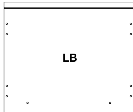
402x340x18mm
