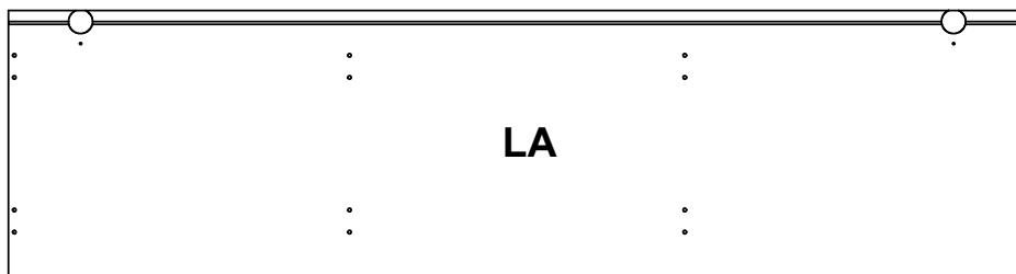
1472x391x15mm
