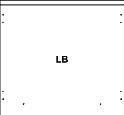
516x481x22mm
